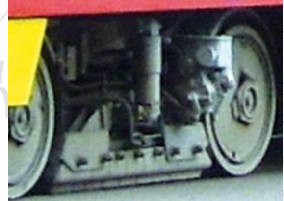
elektromágneses sínfék
